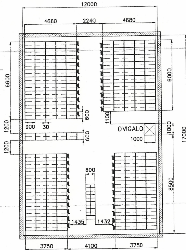
TLOVIS NADSTROPJA
