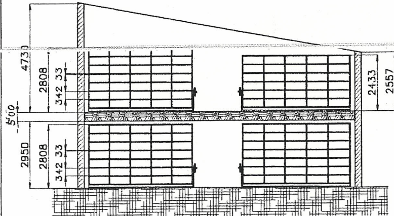
PREREZ A-A
